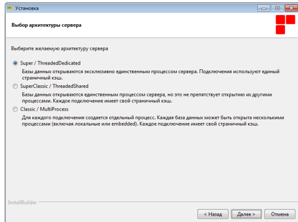
Рис. 4.5 — Выбор архитектуры сервера
