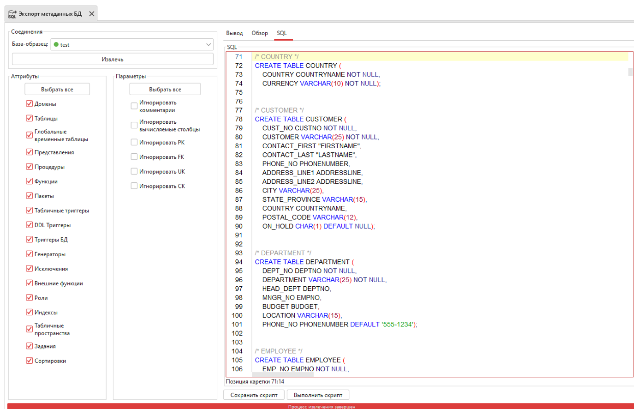
Рисунок 6.4 — Вкладка SQL
