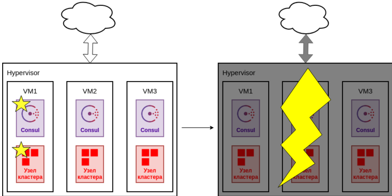
Рис. 7: Сбой гипервизора
