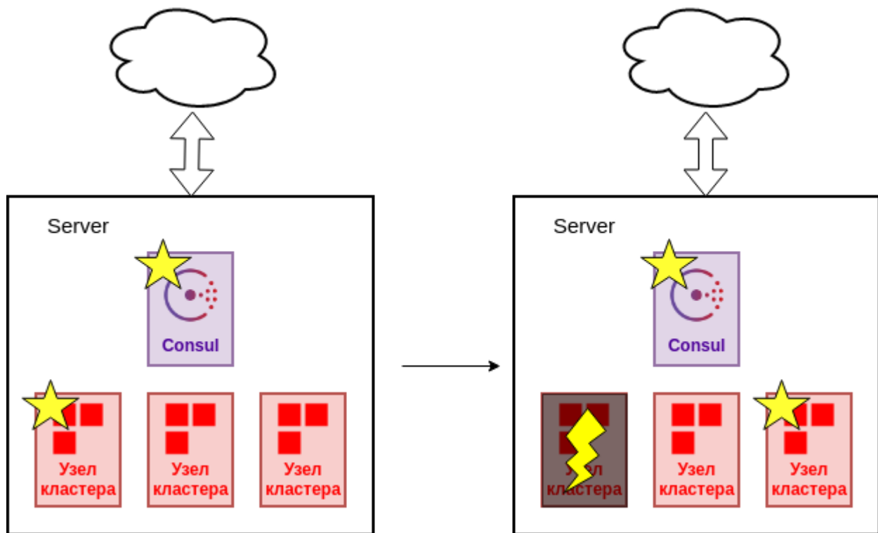
Рис. 4: Сбой процесса
