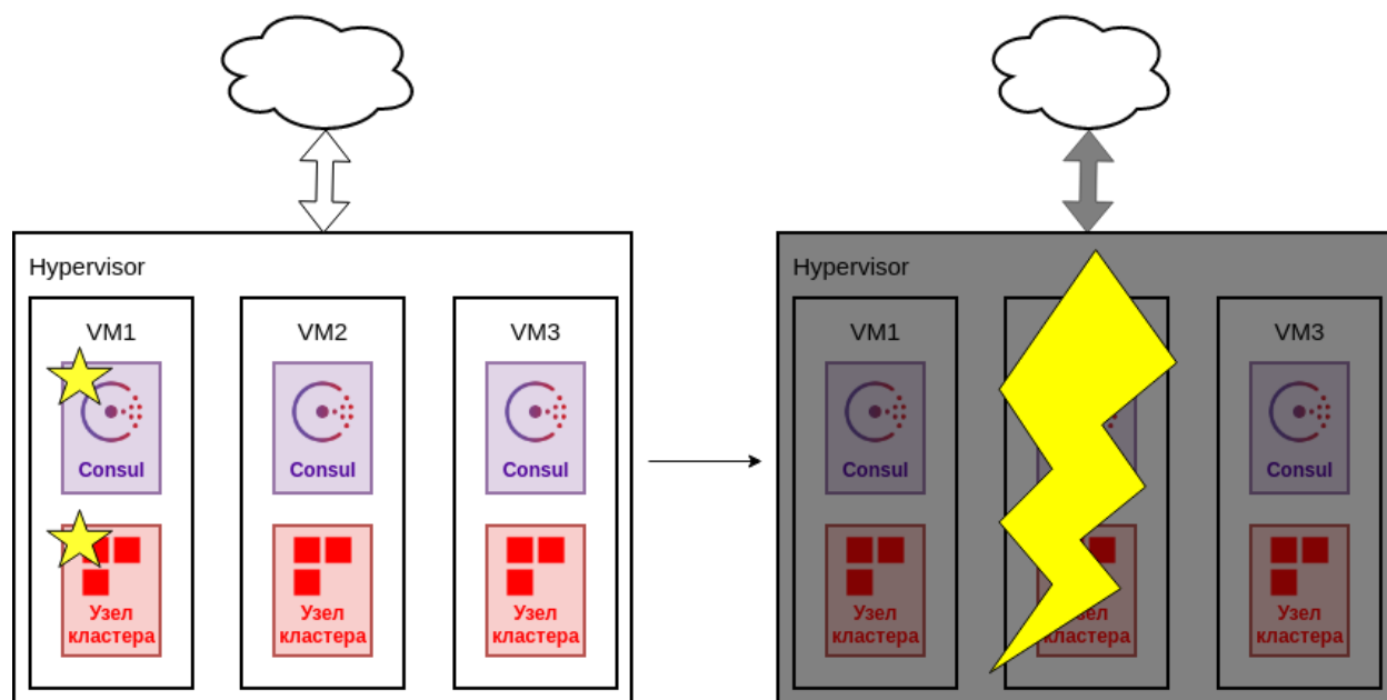
Рис. 7: Сбой гипервизора
