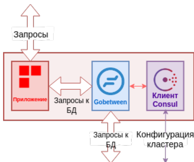
Рис. 3: Схематический вид узла приложения
