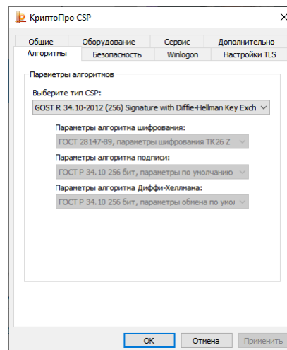
Рисунок 2.1 — Настройка алгоритмов
