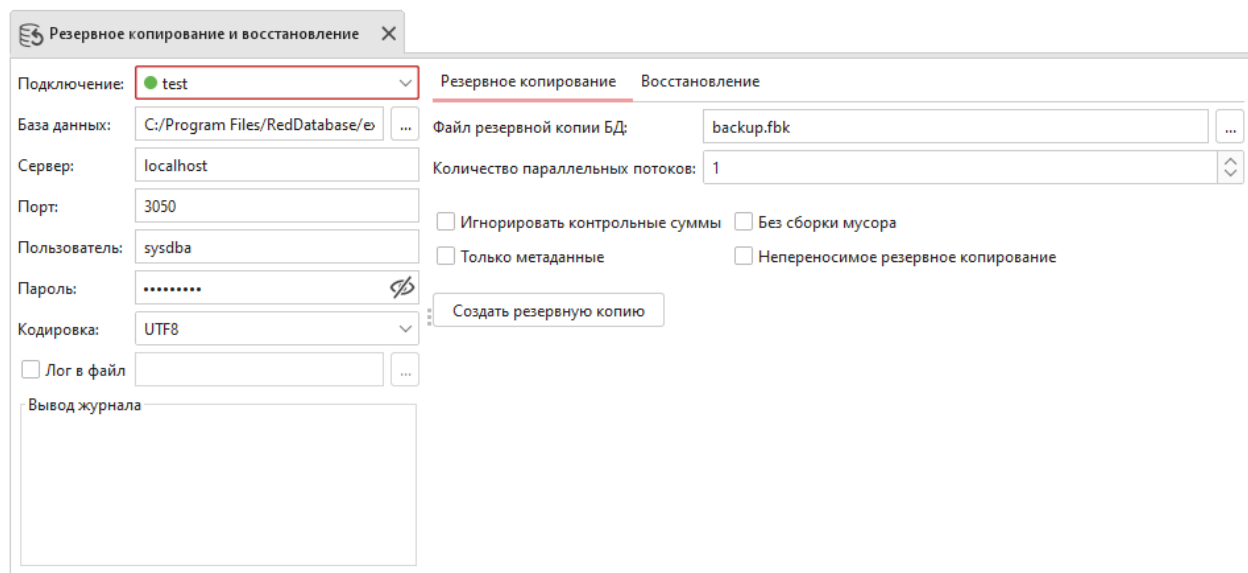
Рисунок 4.12 — Резервное копирование и восстановление
