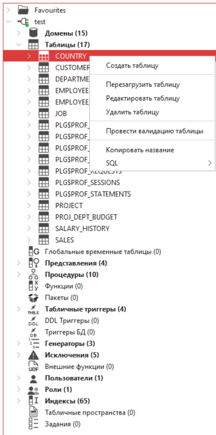
Рисунок 3.3 — Дерево подключений
