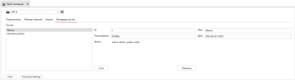
Рисунок 11.4 — Менеджер сессий
