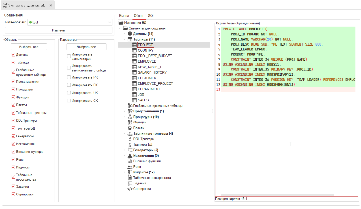
Рисунок 6.3 — Вкладка Обзор
