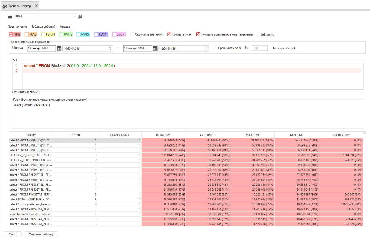
Рисунок 11.3 — Результирующая таблица
