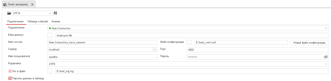
Рисунок 11.1 — Трейс менеджер
