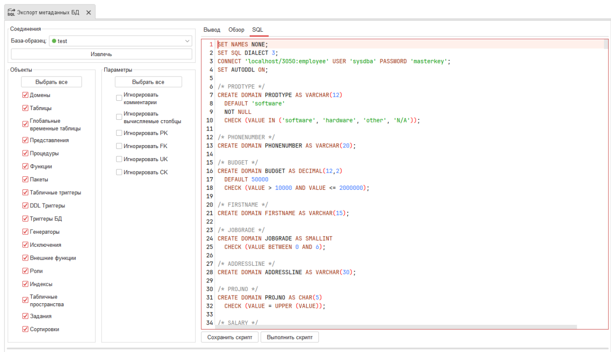
Рисунок 6.4 — Вкладка SQL
