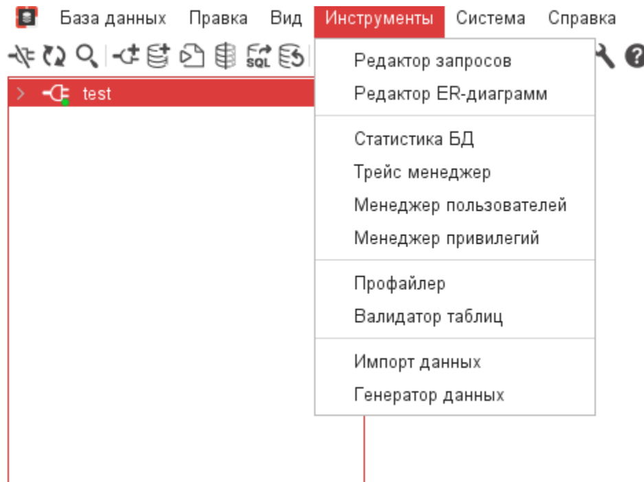
Рисунок 7.1 — Вкладка Инструменты
