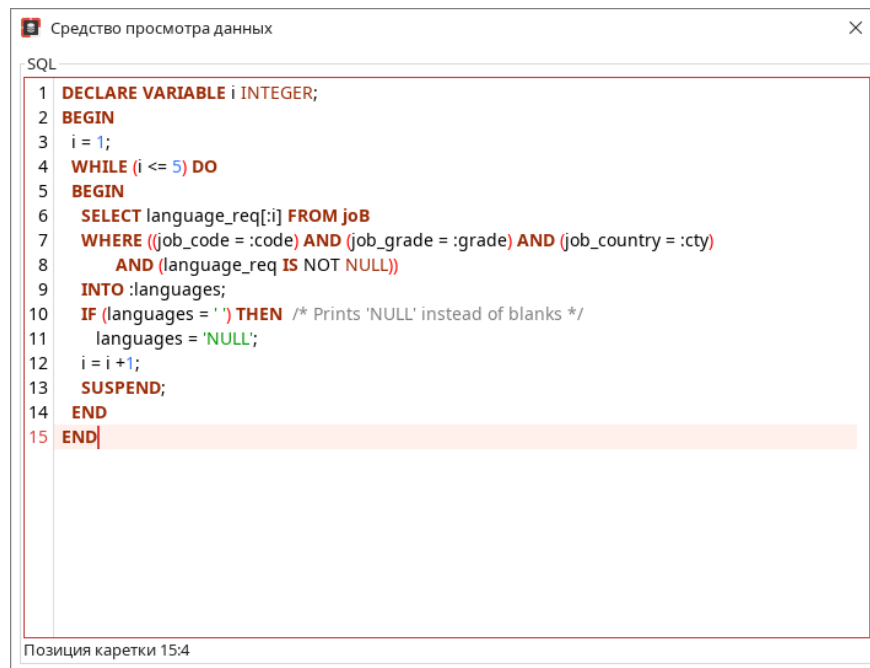
Рисунок 14.4 — Окно просмотра данных
