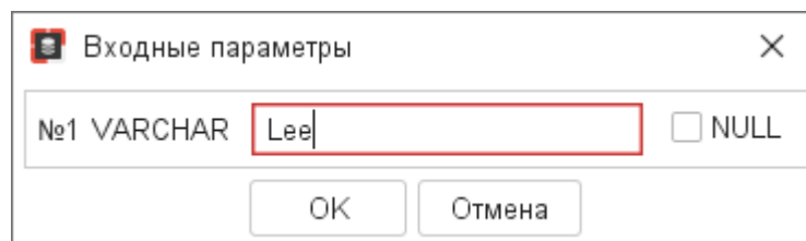
Рисунок 8.3 — Неименованный параметр
