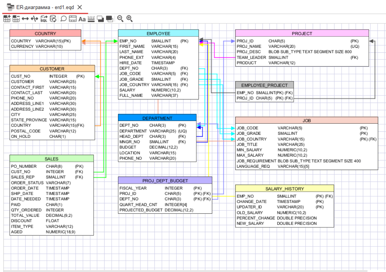
Рисунок 9.1 — Редактор ER-диаграмм
