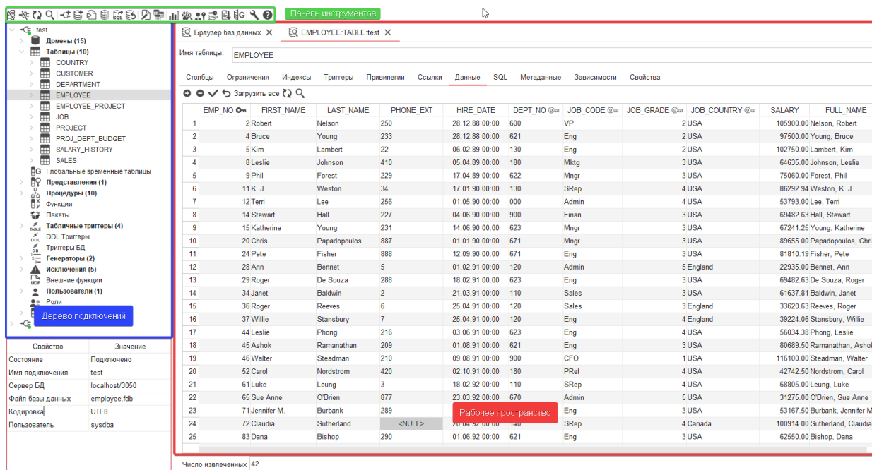
Рисунок 3.1 — Интерфейс приложения
