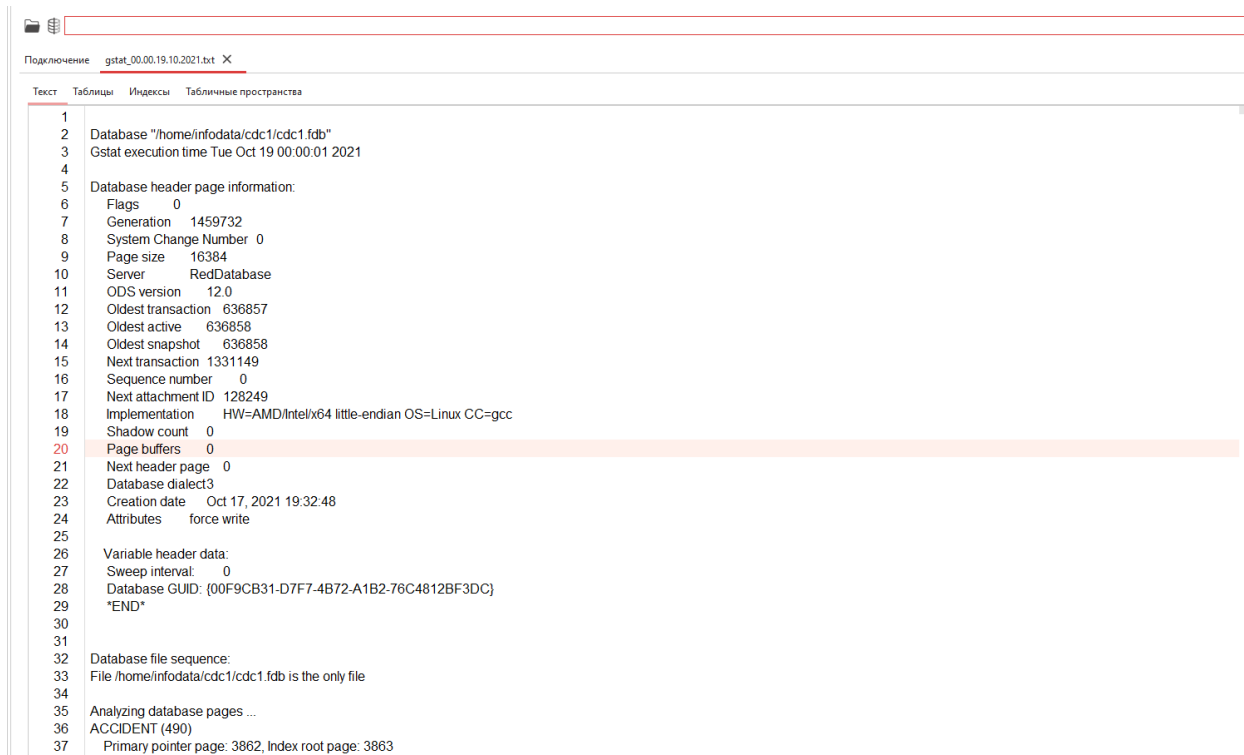
Рисунок 10.2 — Собранная статистика
