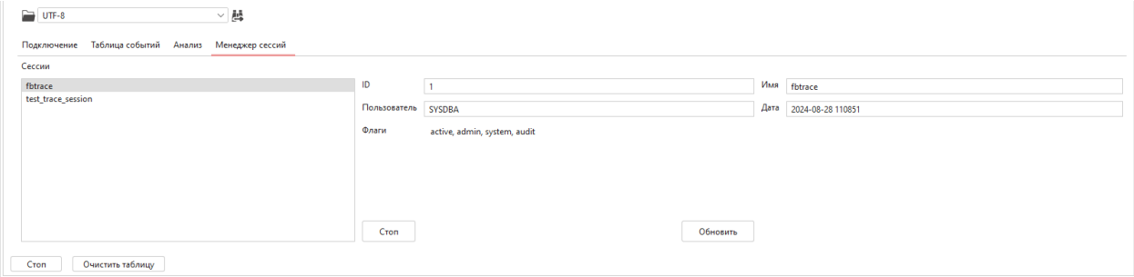
Рисунок 11.7 — Менеджер сессий
