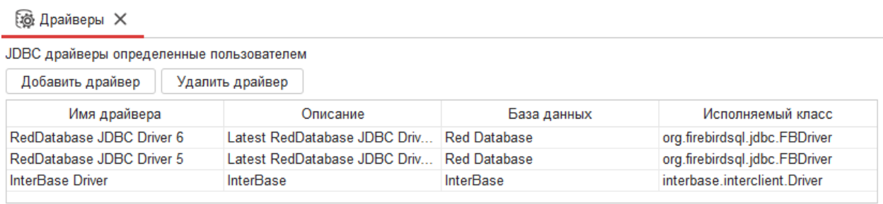
Рисунок 18.1 — Драйверы
