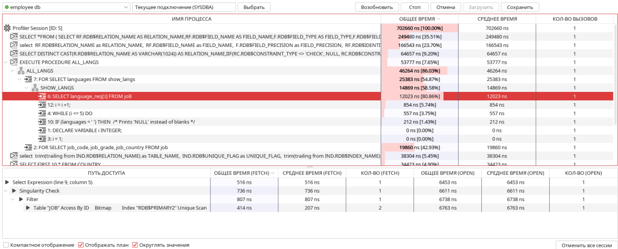
Рисунок 14.1 — Профайлер
