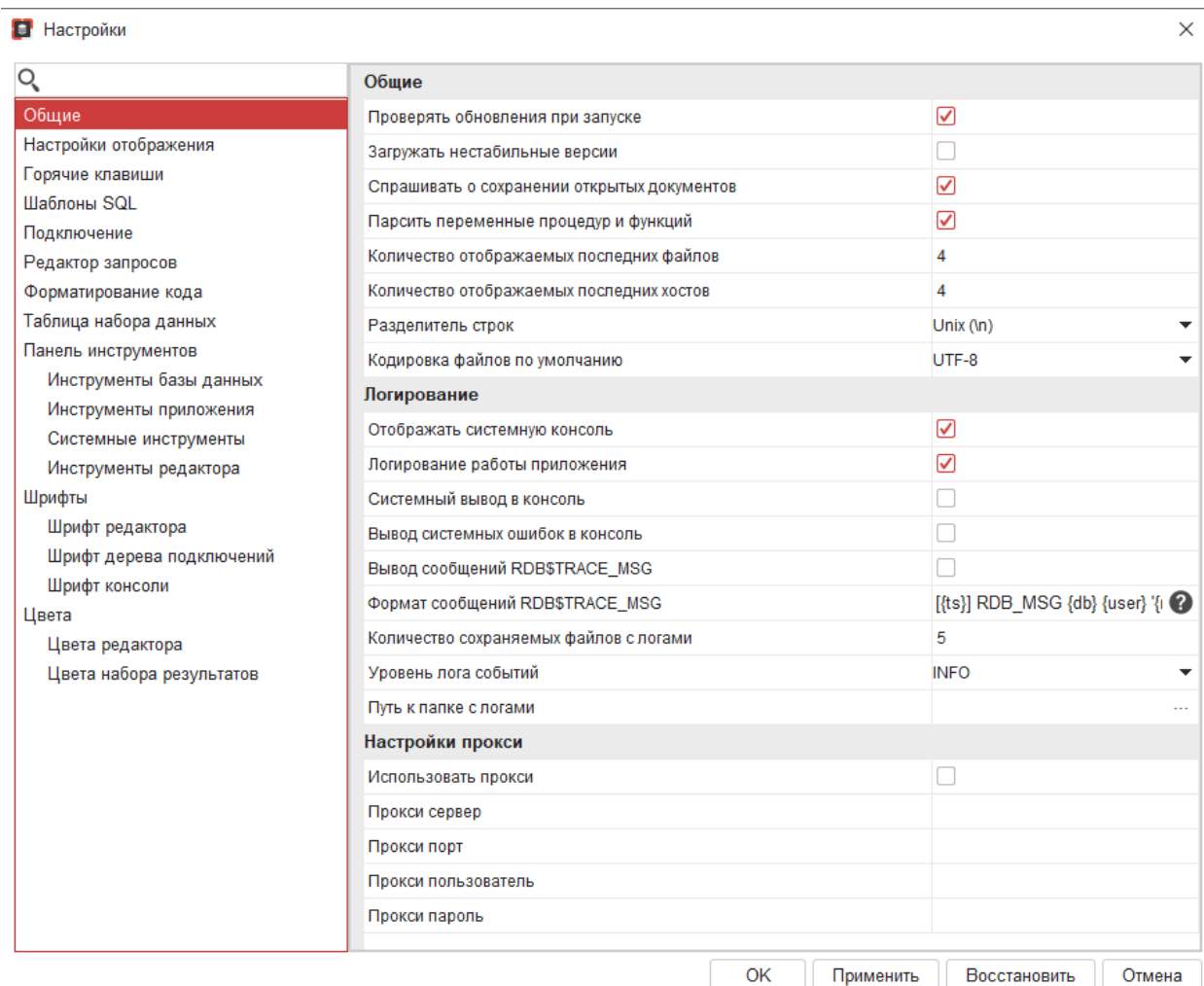
Рисунок 18.4 — Настройки
