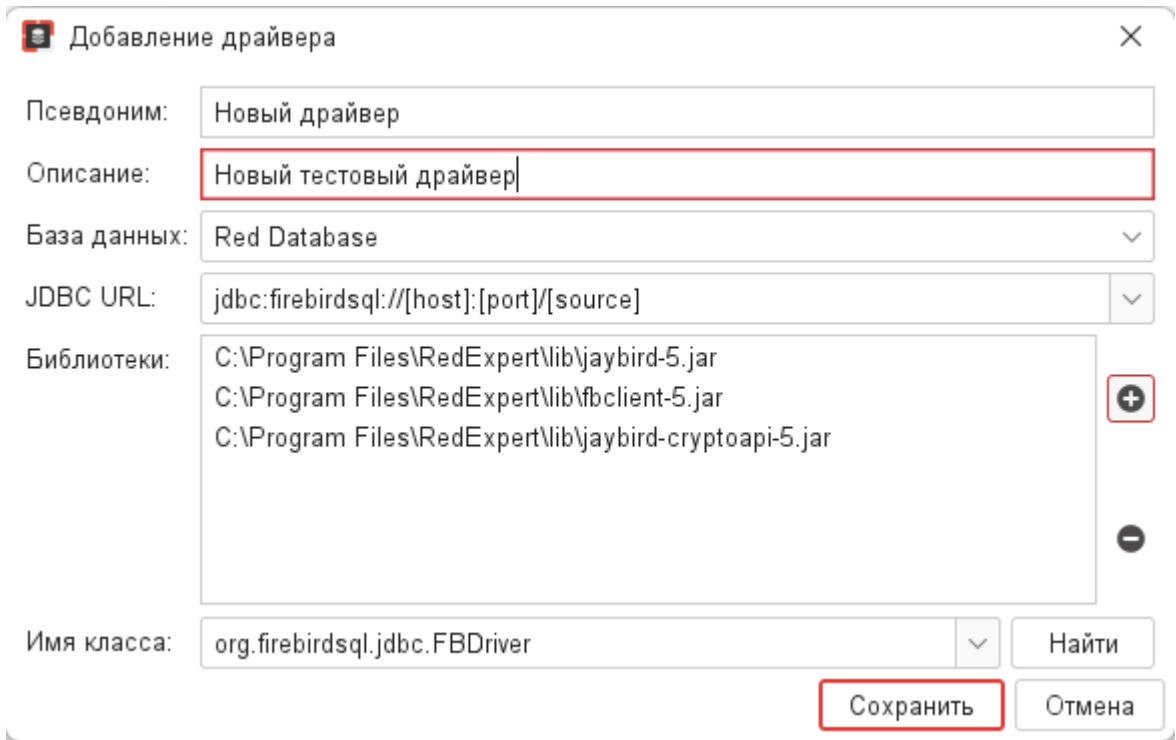
Рисунок 18.2 — Добавление драйвера
