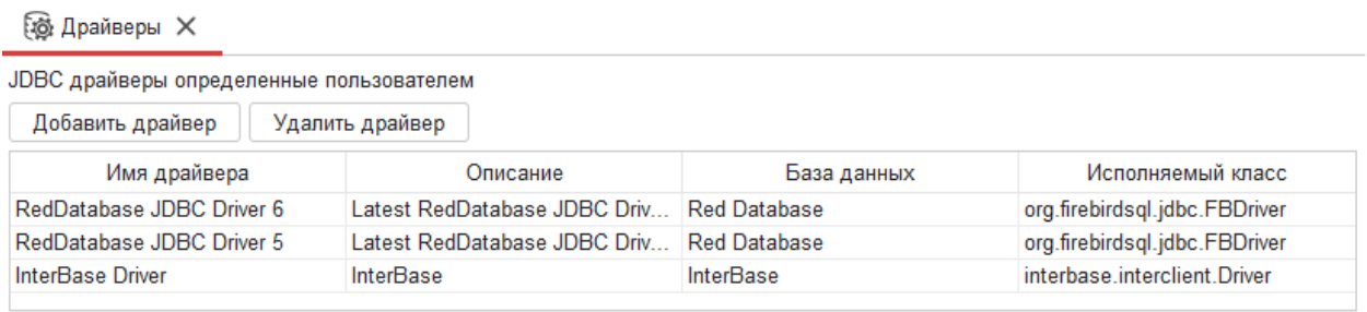
Рисунок 18.1 — Драйверы
