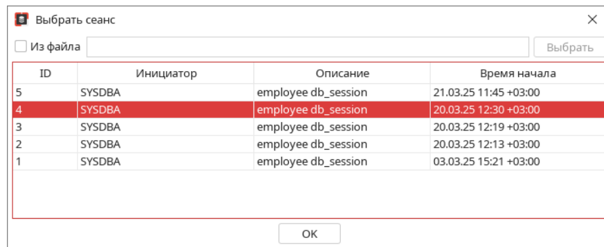
Рисунок 14.3 — Сохранённые сессии
