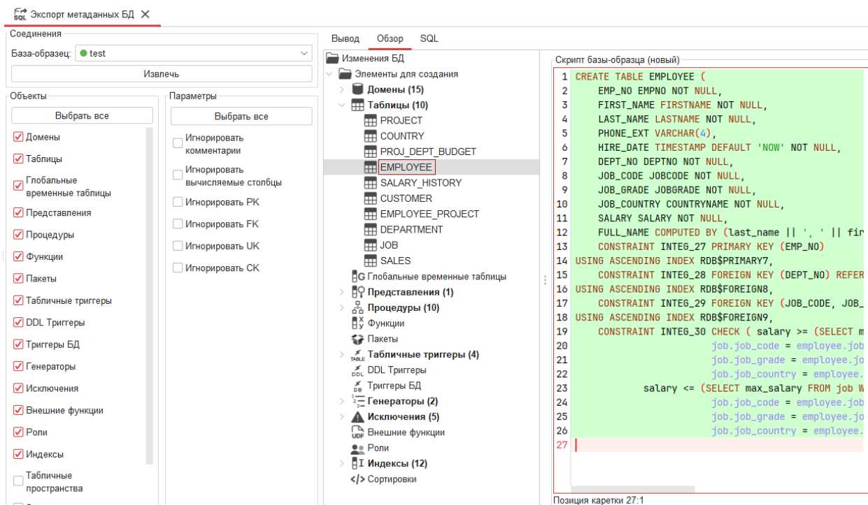
Рисунок 6.1 — Экспорт метаданных
