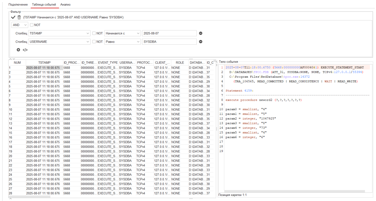
Рисунок 11.4 — Таблица событий
