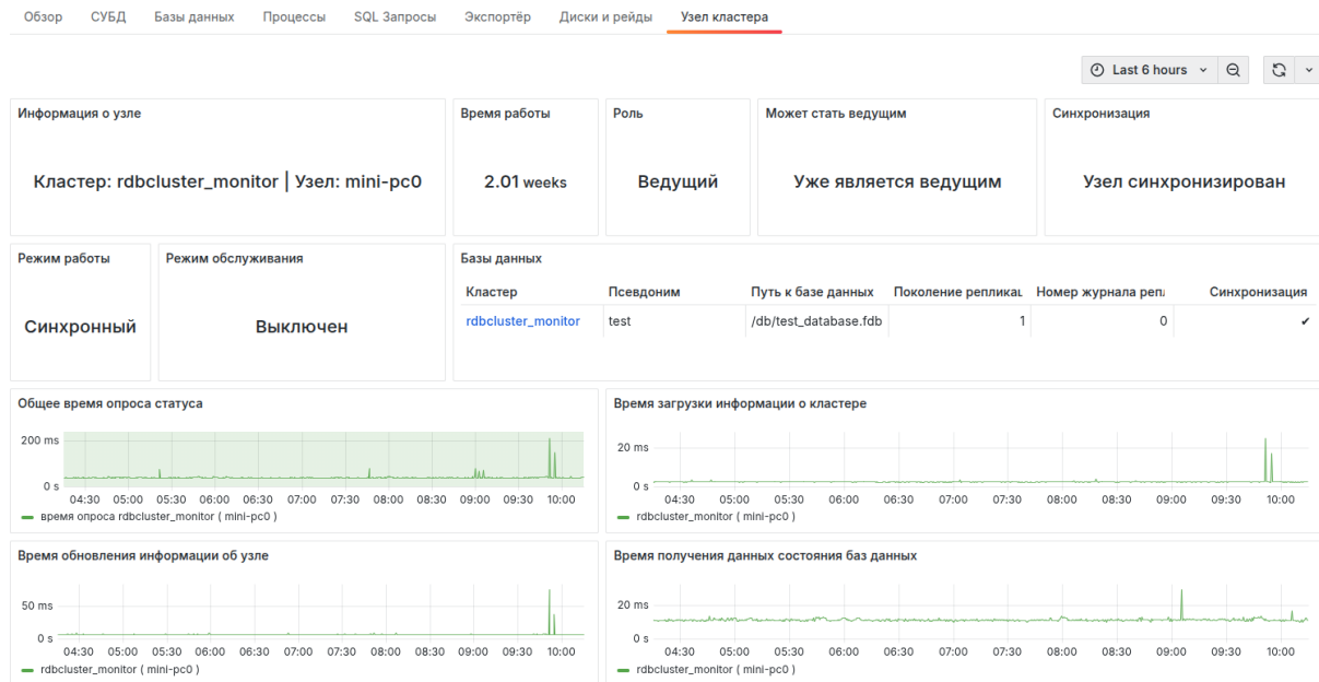
Рисунок 5.28 — Информация об узле кластера
