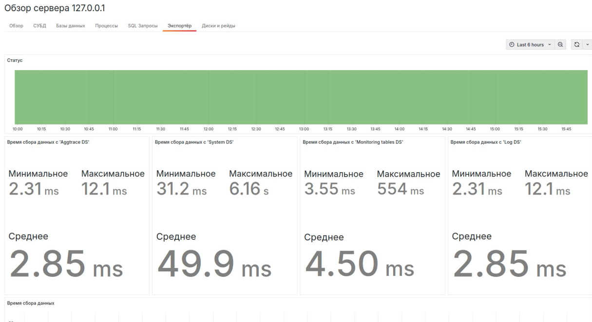
Рисунок 5.22 — Экспортёр
