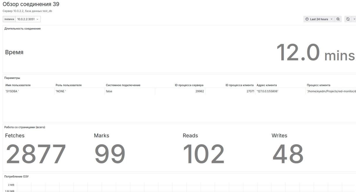
Рисунок 5.16 — Обзор соединения
