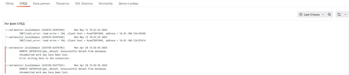
Рисунок 5.6 — Лог СУБД
