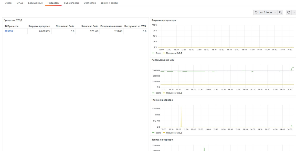
Рисунок 5.19 — Процессы СУБД
