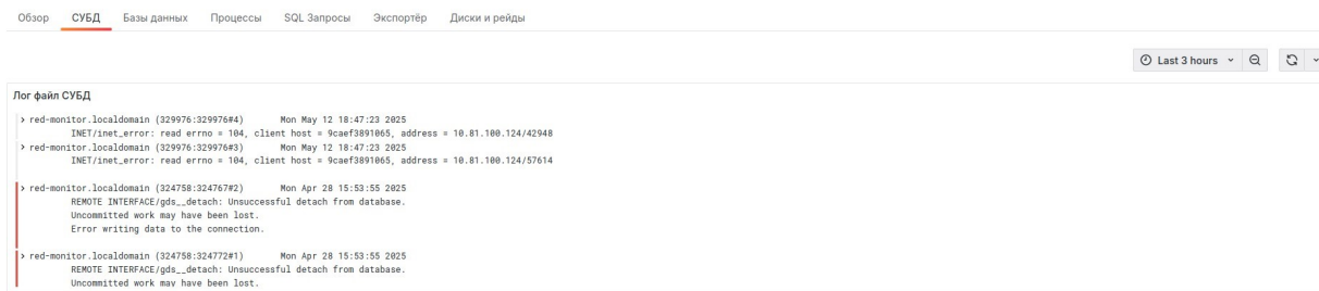
Рисунок 6.6 — Лог СУБД
