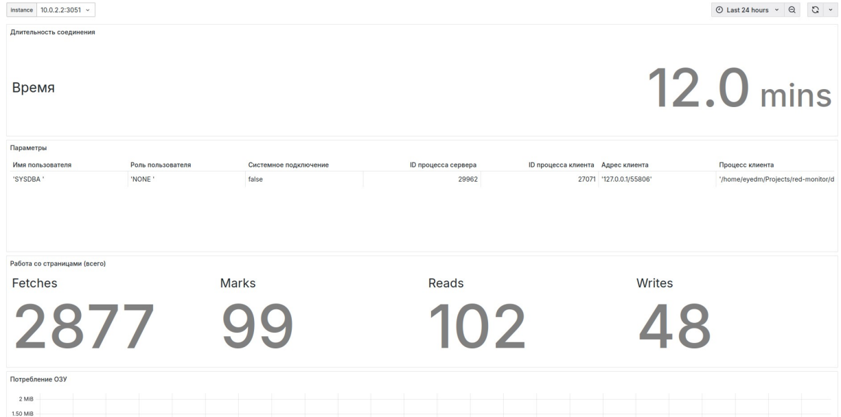
Рисунок 6.16 — Обзор соединения
